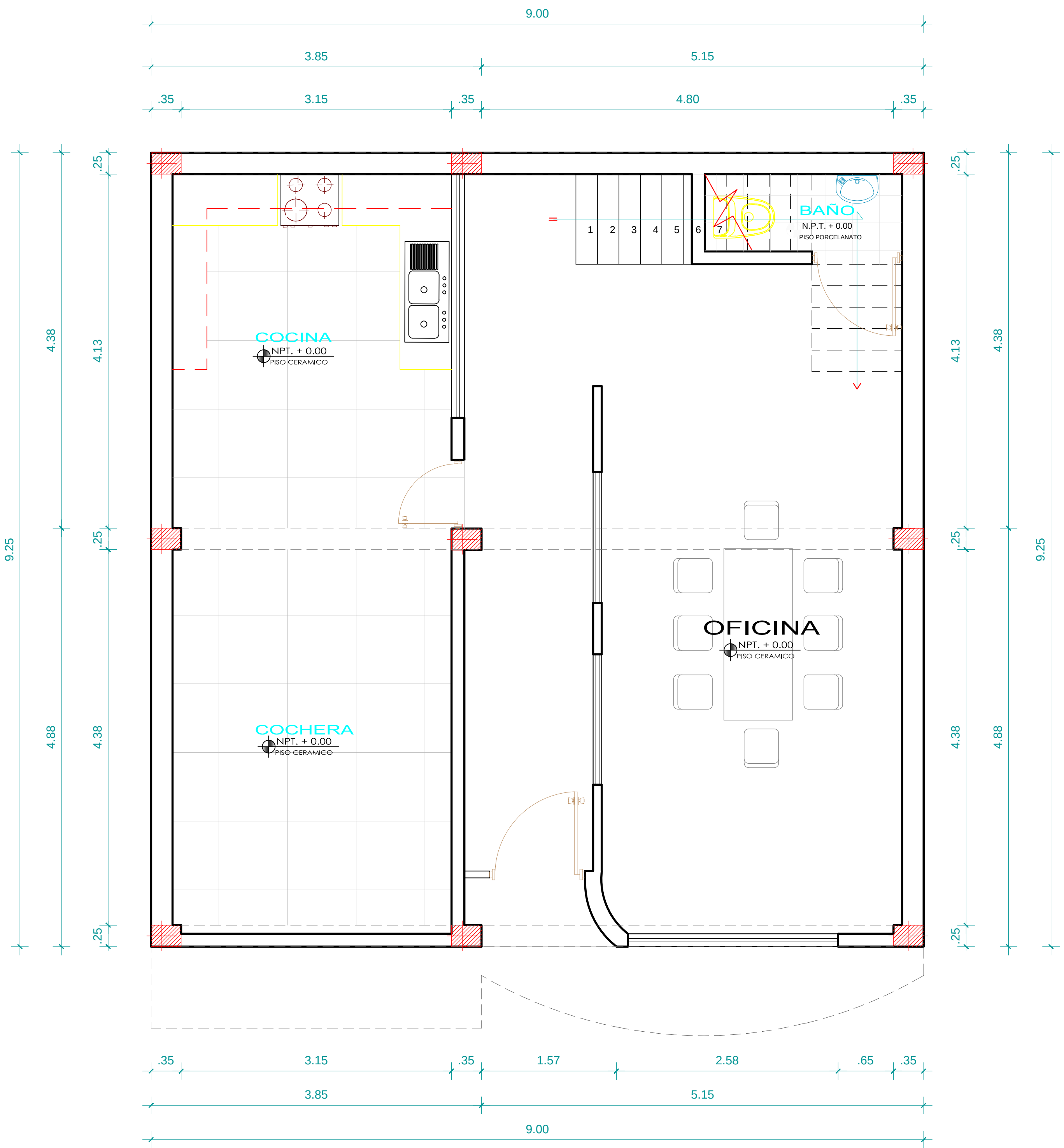
1 PLANTA PRIMER NIVEL ESC:1/50
