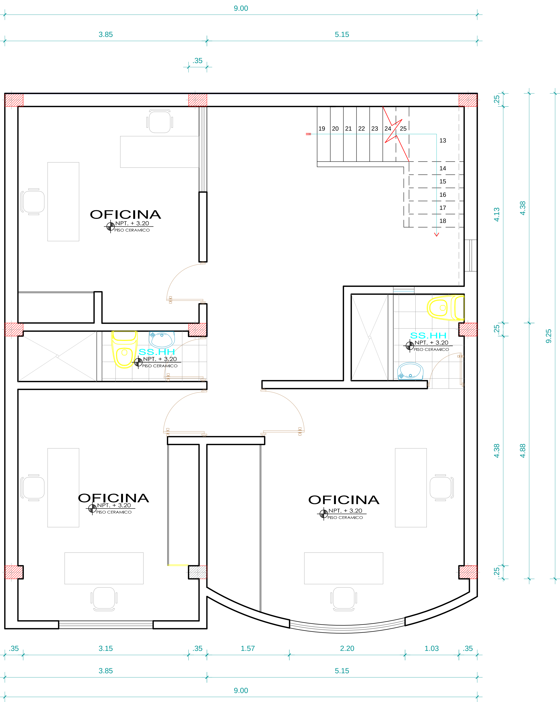
1 PLANTA SEGUNDO NIVEL ESC:1/50
